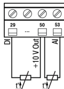
Рисунок 6.13 – Подключение термистора*
